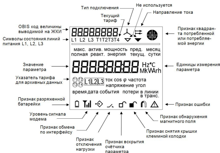
Рисунок 4.1 - Расположение информации на индикаторе абонентского дисплея
